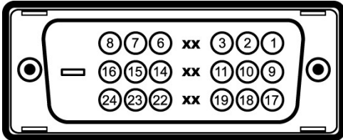
針腳編號 已連接訊號連接線的24針腳端
